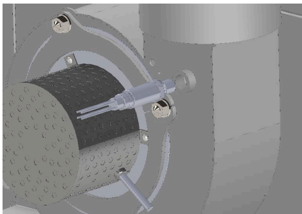
Obrázek 7 Instalace lambda sondy do odtahového ventilátoru
