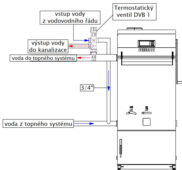
Obrázek 8 Zapojení samočinného dochlazování
