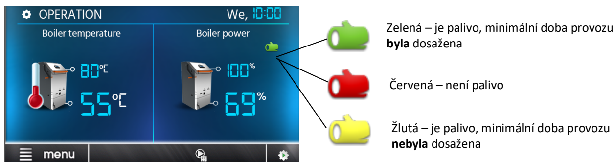
Obrázek 9. Barevné zobrazení signalizace paliva
